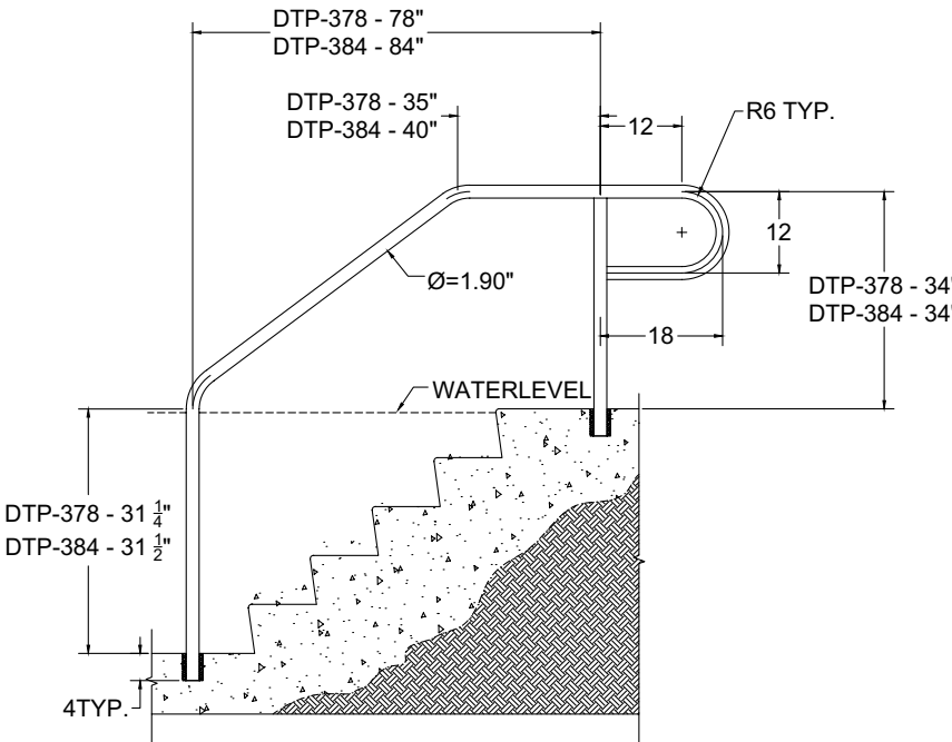
ADA DTP-3 BEND
