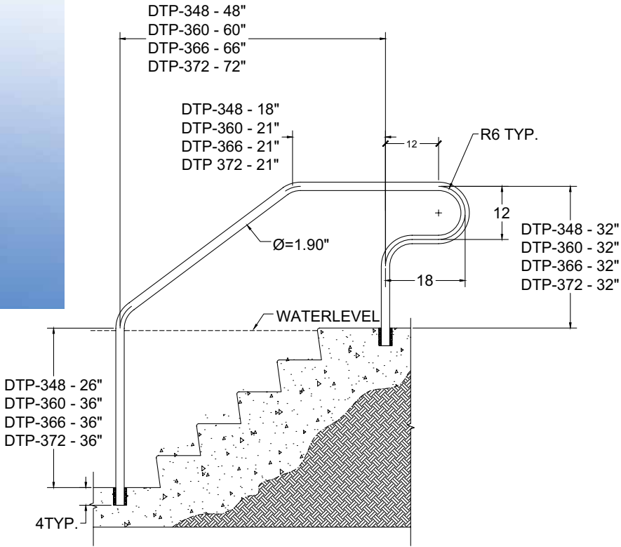
ADA DTP-3 BEND
